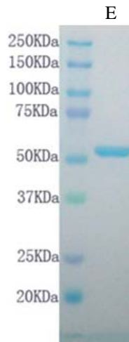
E: GST-NS3 (HCV/Genotype-2b/Con)
